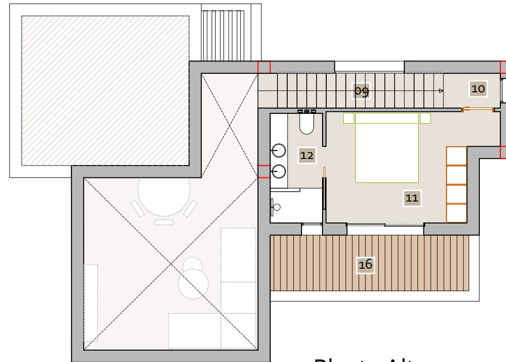
Planta Alta
